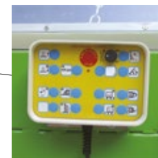
Panel de mandos eléctrico con sistema de regulación de la velocidad de la lona de descarga y botón de emergencia de parada de la máquina
