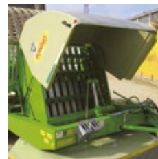
Bastidor de fibra de vidrio con sistema de apertura para acceso a la zona de la cinta transportadora autocargadora
