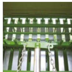
Cinta transportadora autocargadora L: 1400 mm - 8/9/10 portadores con descarga facilitada. Predisposición 9 cuchillas cortahierba
